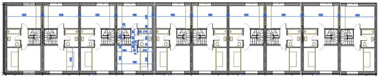
1 этаж
