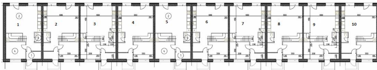
План 1 этажа
