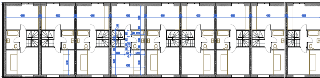
План 2 этажа
