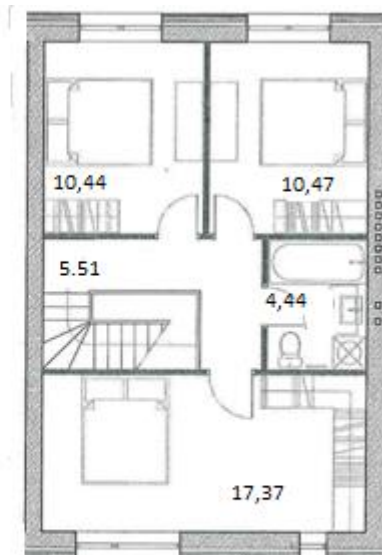
План 2 этажа
