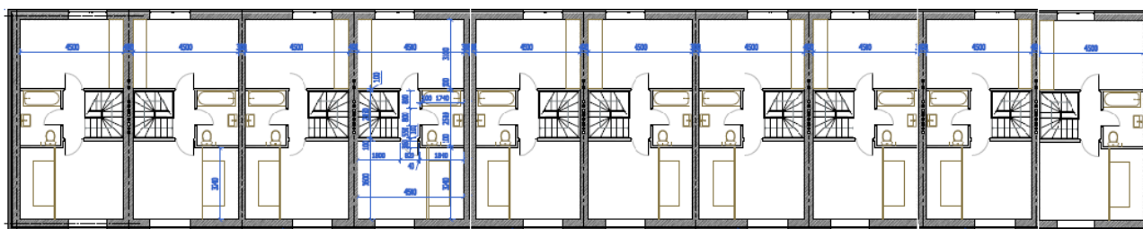
План 2 этажа
