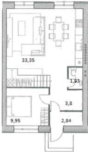
План 1 этажа
