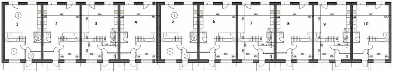
План 1 этажа
