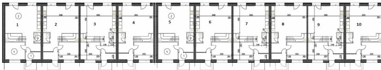
План 1 этажа
