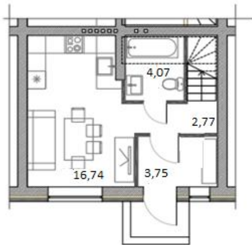
План 1 этажа
