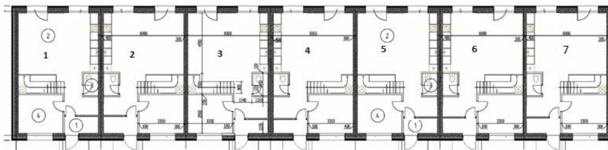
План 1 этажа
