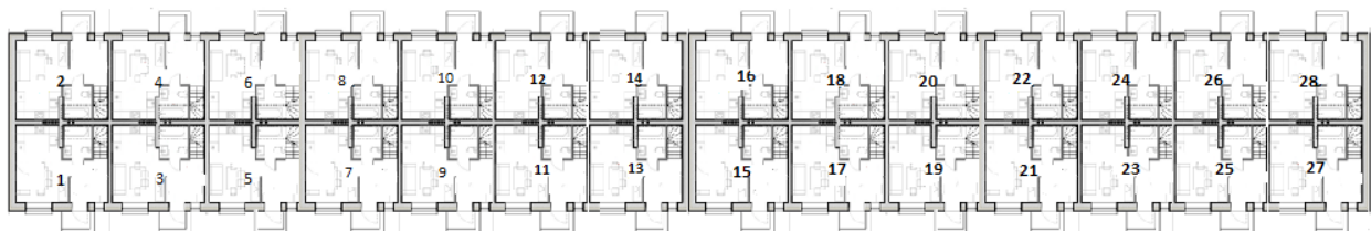
План 1 этажа
