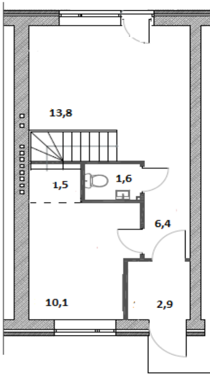
План 1 этажа
