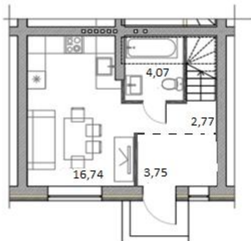
План 1 этажа
