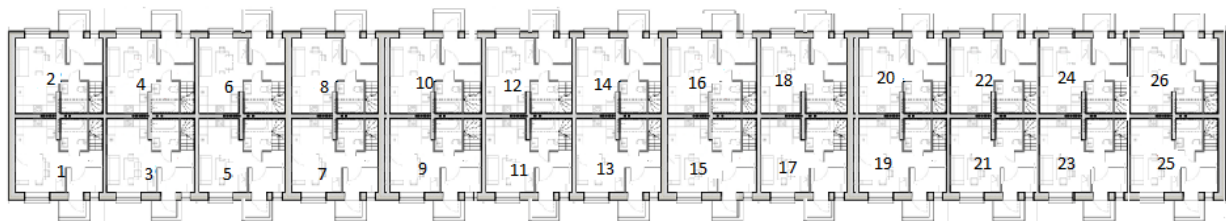
План 1 этажа
