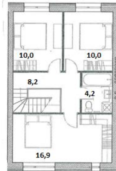
План 2 этажа
