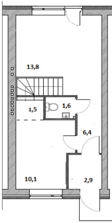
План 1 этажа
