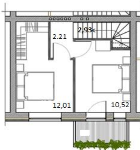
План 2 этажа
