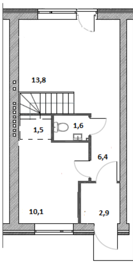
1 этаж
