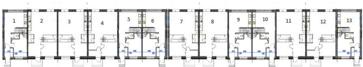
План 1 этажа
